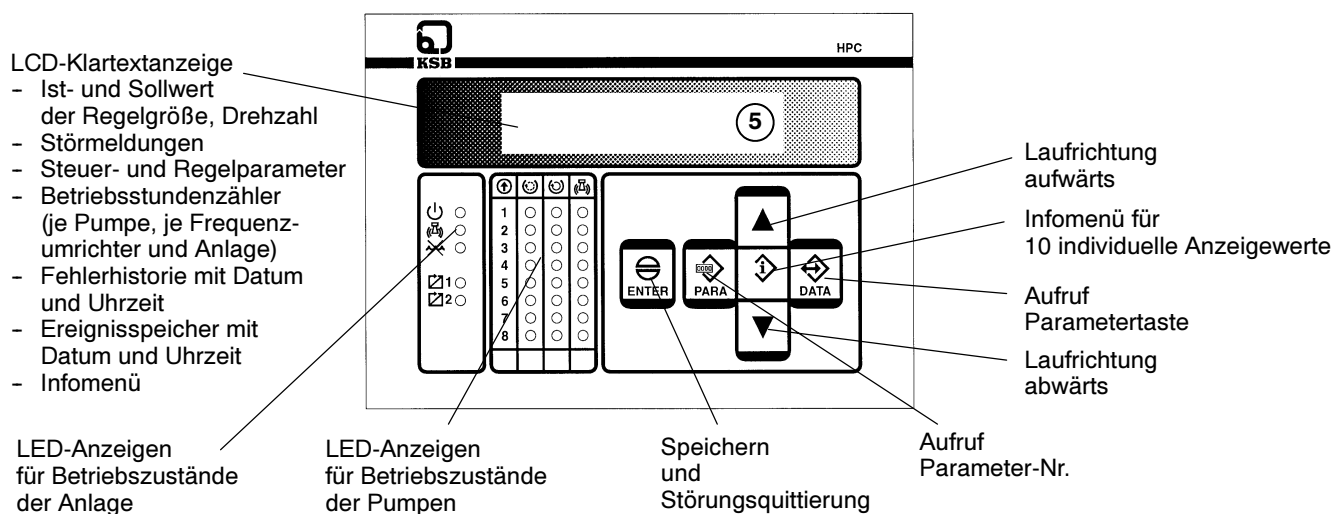
Ausführungsbeispiel Wandmontage
