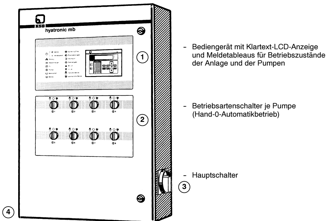
Ausführungsbeispiel Wandmontage
